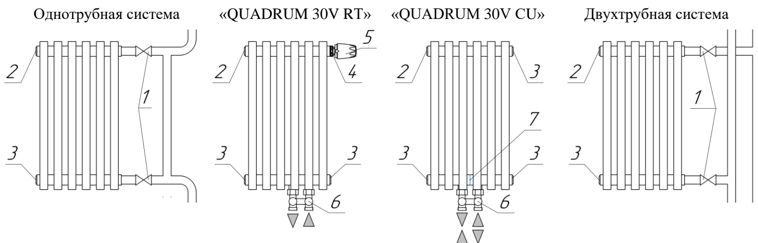
Рис.2 1. Вентиль. 2. Кран Маевского - воздухоотводчик. 3. Пробка глухая. 4. Встроенный термокран. 5. Термостатический элемент. 6. Запорно-присоединительный клапан нижнего подключения. 7. Внутренняя перегородка.
